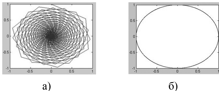
Рис. 3. Графики зависимости y_2 от y_1 (метод Рунге-Кутты с шагом дискретизации 0,5) без коррекции (а) и с коррекцией (б)
