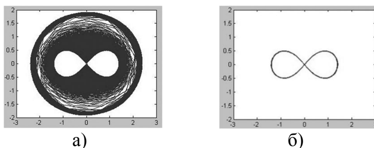
Рис. 4. Графики зависимости y_2 от y_1 (метод Dormand-Prince с шагом дискретизации 0.05, u_1 = 1 ) без коррекции (а) и с коррекцией (б)
