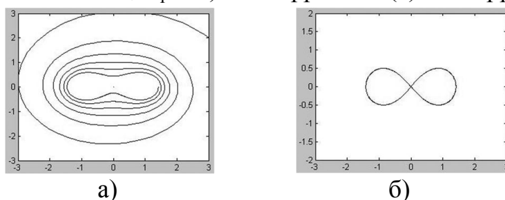
Рис. 5. Графики зависимости y_2 от y_1 (метод Эйлера с шагом дискретизации 0.5, u_1 = 0.01 ) без коррекции (а) и с коррекцией (б)
