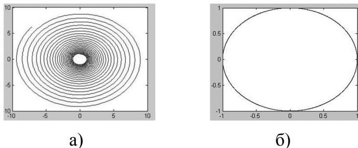
Рис. 2. Графики зависимости y_2 от y_1 (метод Эйлера с шагом дискретизации 0.5) без коррекции (а) и с коррекцией (б)
